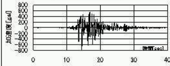
耐震時2階応答加速度
